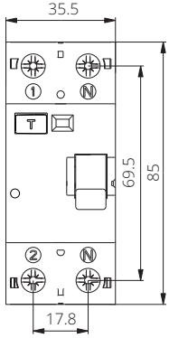
FI2BK ( I_n = 25 - 80\text{ A} )
