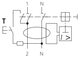
FI2, FI2K, FI2S, FI2F
