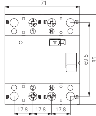
FI2BK ( I_n = 100 - 125\text{ A} )
