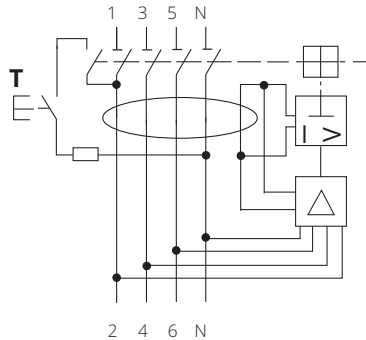
NF14BK, NF14BS
