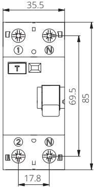
FI2, FI2K FI2S, FI2F
